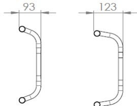
HUM030403 & HUM030404 Barra standar de respaldo Oval y barra más alejada
